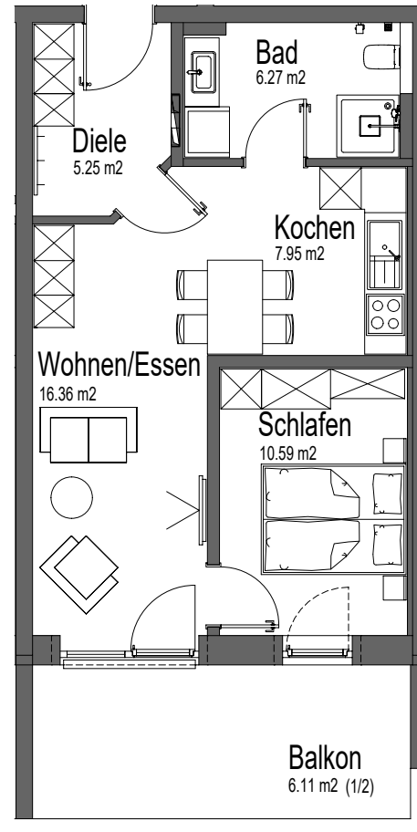
Wohnung 7 Haus E 52.524 m 2
