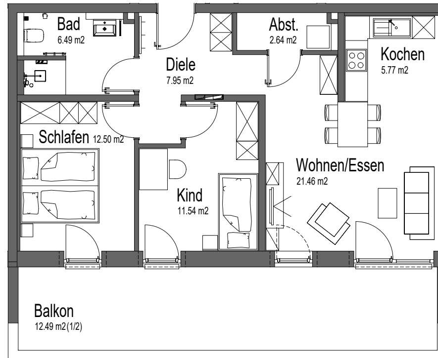
Wohnung 5 Haus D 80.834 m 2
