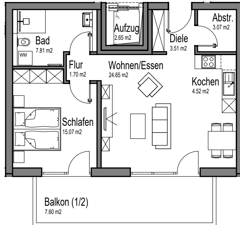
Wohnung 5 67.939 m 2
