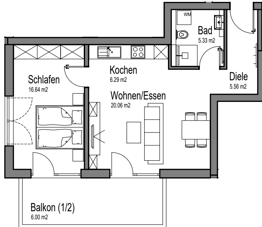
Wohnung 6 59.890 m 2
